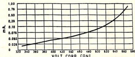
Assorbimento di corrente per \mu\text{F} in funzione della tensione in un condensatore della Serie 3900.
