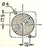
Foratura telaio
