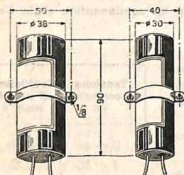
Serie per fissaggio orizzontale mediante fascetta.
