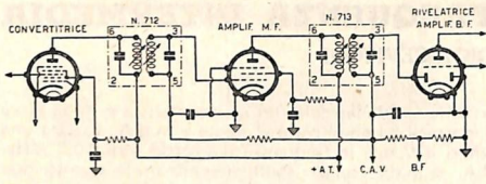
Esempio tipico di impiego della serie 711
