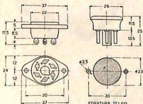
N. 493 - N. 494 - N. 498 Ingombro e foratura del telaio.
