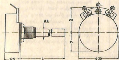
Dimensioni d'ingombro dei potenziometri a grafite senza interruttore.
