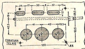
Foratura del telaio
