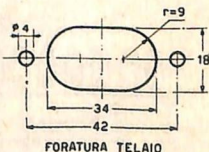
FORATURA TELAIO
