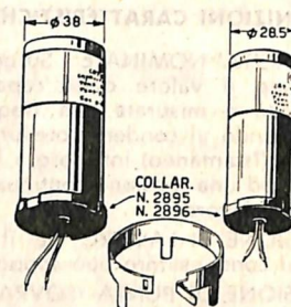
Serie per fissaggio orizzontale (mediante fascetta) o verticale (mediante collarino).
