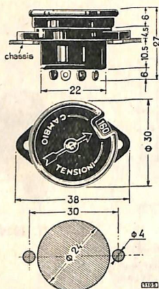
Foratura chassis Mod. 1044 - 45 - 46.
