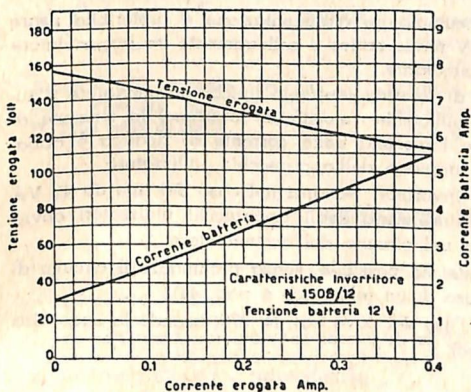
N. 1508/12 - Tensione alternata erogata in funzione della corrente continua assorbita.
