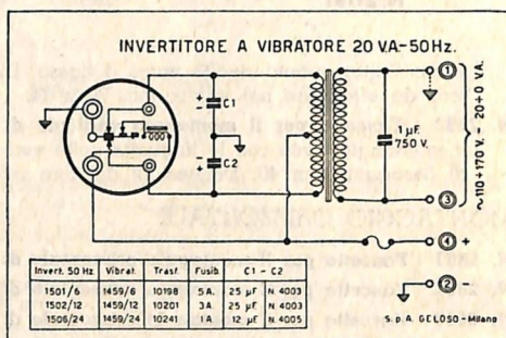
Schema invertitore 20 VA.
