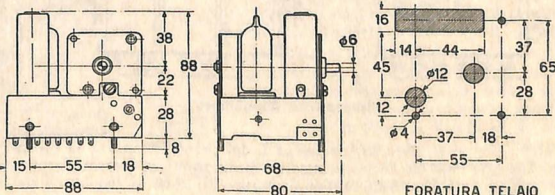
FORATURA TELAIO
