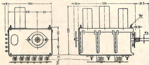
Dimensioni d'ingombro
