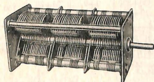
Condensatore variabile triplo (N. 773) della Serie 770
