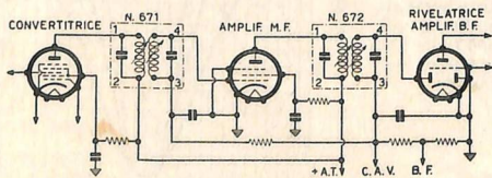
Esempio tipico di impiego: numerazione e corrispondenza dei terminali.
