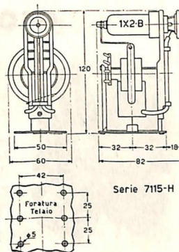
Dimensioni d'ingombro e foratura del telaio del trasformatore orizzontale N. 7115/H.
