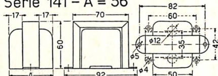
Serie 2121 - A = 65 Foratura telaio (1)
