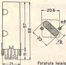
Foratura telaio
