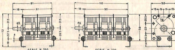
Condensatore variabile triplo (N. 773) della Serie 770
