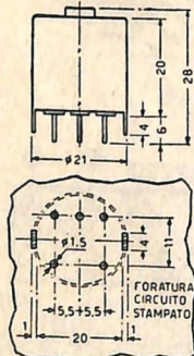
Ingombro e foratura serie N. 1151
