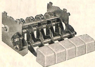
N. 181 - Tastiera di comando a 5 tasti e 5 posizioni, con interruttore di rete (esempio delle combinazioni: interruttore - fono - gamma 1 - gamma 2 - gamma 3; vedi esempio d'impiego nel G 332). Tasti in materia plastica colore bianco avorio. Le dimensioni d'ingombro sono indicate qui sotto. Peso netto circa gr 300.
