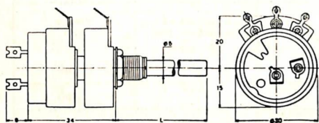
Dimensioni d'ingombro dei potenziometri doppi a perno unico.
