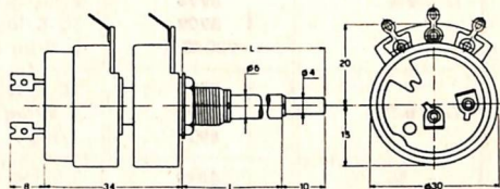
Dimensioni d'ingombro dei potenziometri doppi a due perni indipendenti.
