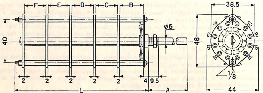
Dati d'ingombro dei commutatori serie 2000.
