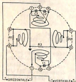
Schema del N. 7215/D
