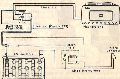
Inserimento di un interruttore generale a relè.
