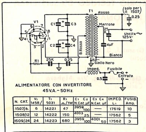
Schema invertitore 45 VA.
