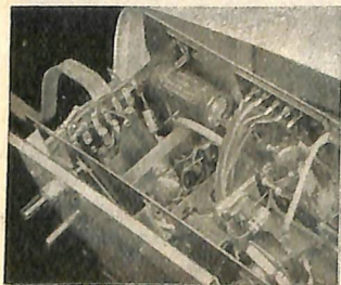
Particolare del collegamento all'entrata antenna 300 ohm del sintonizzatore.
