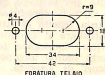
FORATURA TELAIO
