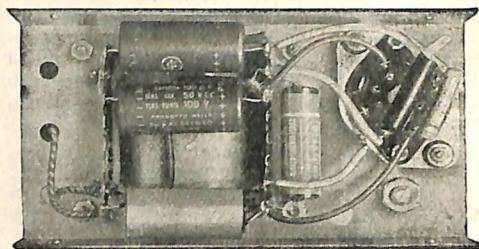
Invertitore 45 VA - Vista dell'interno, sotto al telaio.
