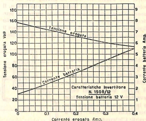
Invertitore N. 1508/12 - Tensione erogata in funzione della corrente fornita e relativa corrente continua assorbita, con carico resistivo.
