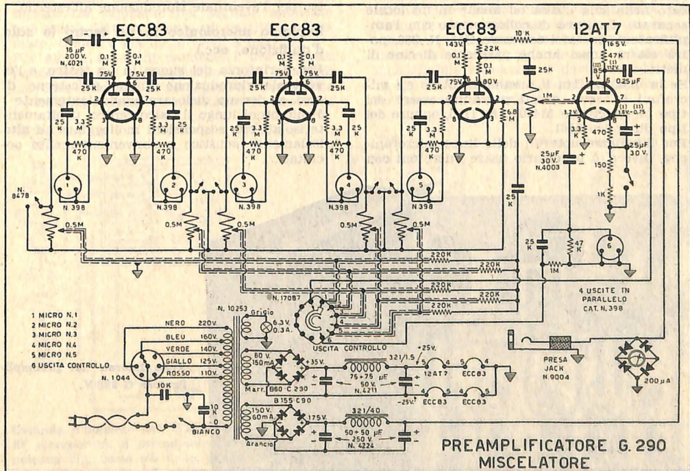
Schema elettrico del G 290-V. Le tensioni agli elettrodi delle valvole sono indicate su lo schema.
