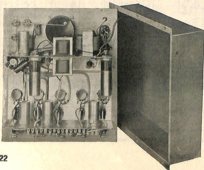
Vista interna del preamplificatore G 290-V.
