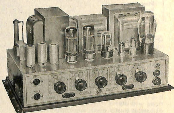
Vista dell'amplificatore G 280 A senza il coperchio.
