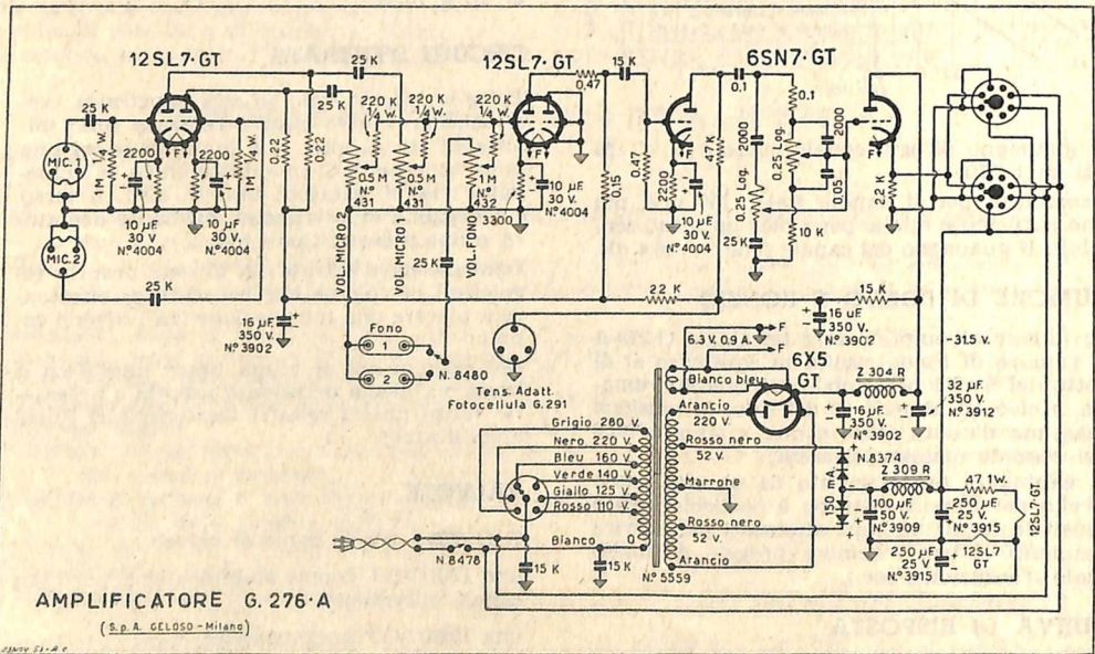
Schema elettrico dell'amplificatore G 276-A
