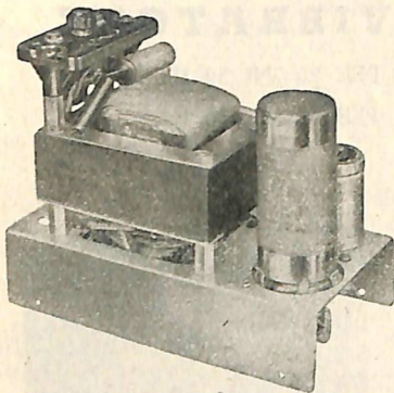
Invertitore 45 VA senza scatola di protezione.
