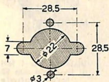
FORATURA TELAIO
