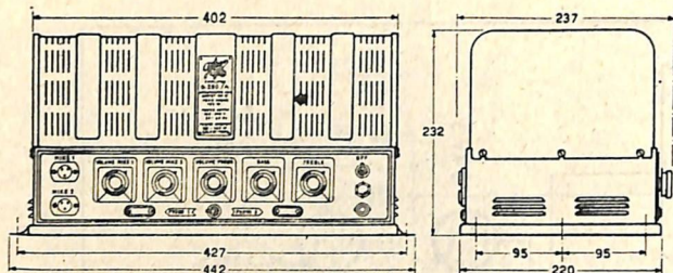
Dimensioni d'ingombro e posizione fori fissaggio - G 280-A.
