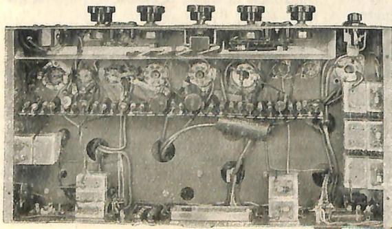
Vista interna del G 280-A.
