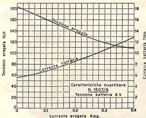
Invertitore N. 1507/6 - Tensione erogata in funzione della corrente fornita e relativa corrente continua assorbita, con carico resistivo.
