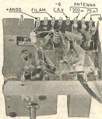
N. 2723 - collegamenti ai terminali.
