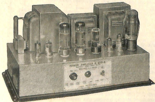
Vista dell'amplificatore di potenza G 279-A senza la copertura traforata.
