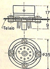
N. 453 - Zoccolo « noval » con supporto elastico, completo di spessori e viti per il montaggio sul telaio portante.
