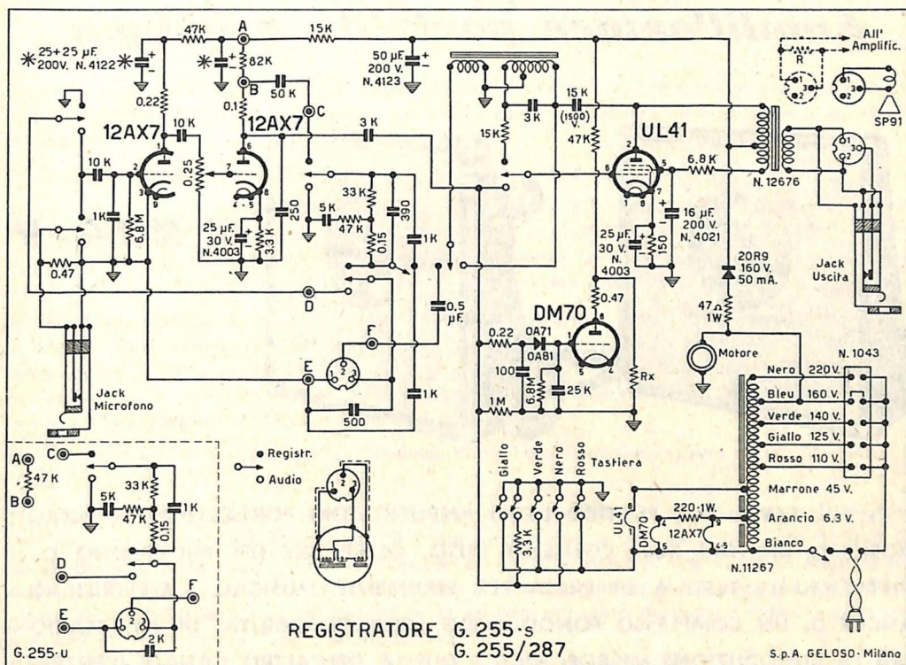
Schema elettrico del magnetofono G. 255/287 - Al posto dell'altoparlante è effettuato il collegamento facoltativo con l'amplificatore di potenza G. 287.
