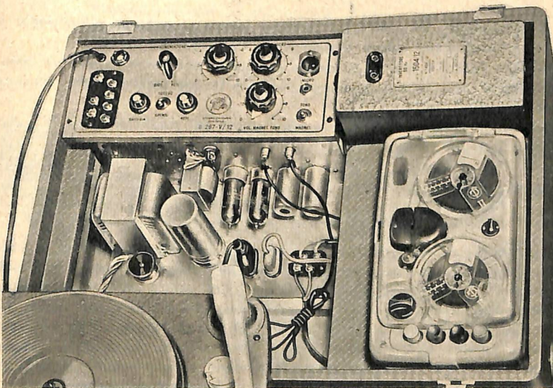
Vista degli attacchi interni del complesso G 287-V. In alto al centro gli attacchi BF del magnetofono e del pick-up, realizzati con due cavetti schermati.
