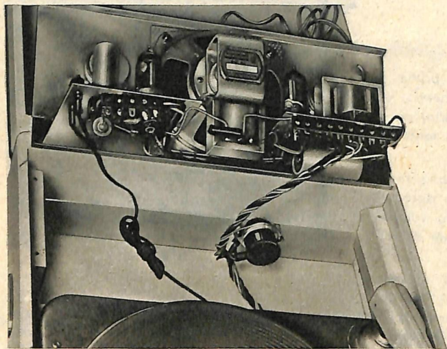
Vista degli attacchi interni della valigetta G 285-V.
