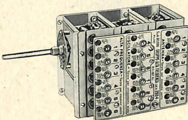
Gruppo di Alta Frequenza Mod. 2616
