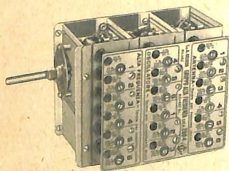
Gruppo per Alta Frequenza N. 2604
