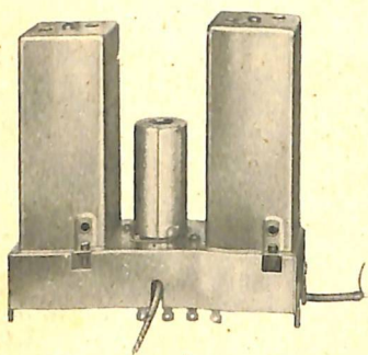
Telaio premontato Mod. 2607 per seconda conversione di frequenza
