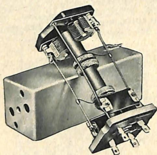
Trasformatore a Media Frequenza
