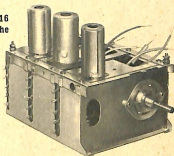
Telaio premontato Mod. 2607 per seconda conversione di frequenza
