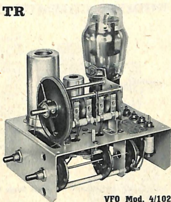
VFO Mod. 4/102
