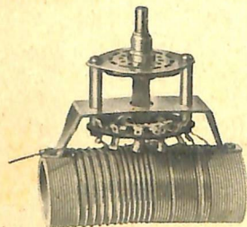
Bobina Mod. 4/110 con commutatore
