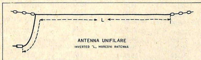
Fig. 5.1 - Antenna unifilare.
