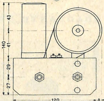
VFO Mod. 4/101
