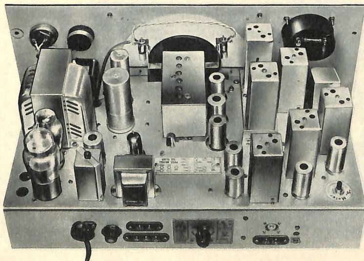
Veduta dello chassis del G 207. Sul retro del telaio si possono osservare, da sinistra a destra: il cambiotioni, il fusibile di rete, la morsettiera a 2 attacchi per l'eventuale collegamento del cavo per il comando « stand-by » a distanza, la morsettiera a 3 attacchi per il collegamento dell'altoparlante, la presa schermata per l'entrata d'antenna ed infine il morsetto di « terra ».
