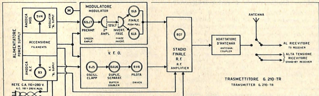
Fig. 3.1 - Schema di principio del trasmettitore G. 210 - Block diagram.
