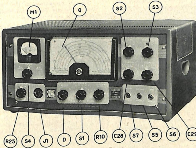
Fig. 4.1 - Vista frontale e nomenclatura organi di comando.
