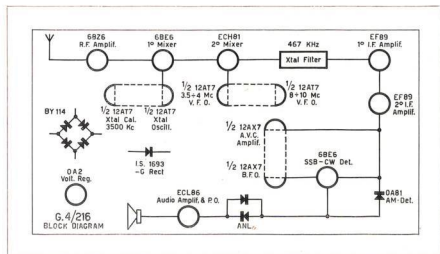
Fig. 1 - G 4/216 - Schema a blocchi
