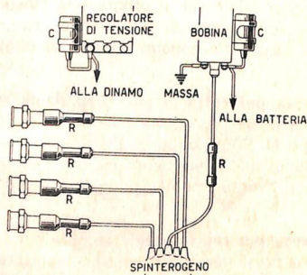
Applicazione dei dispositivi anti-disturbo ad un motore a scoppio.
